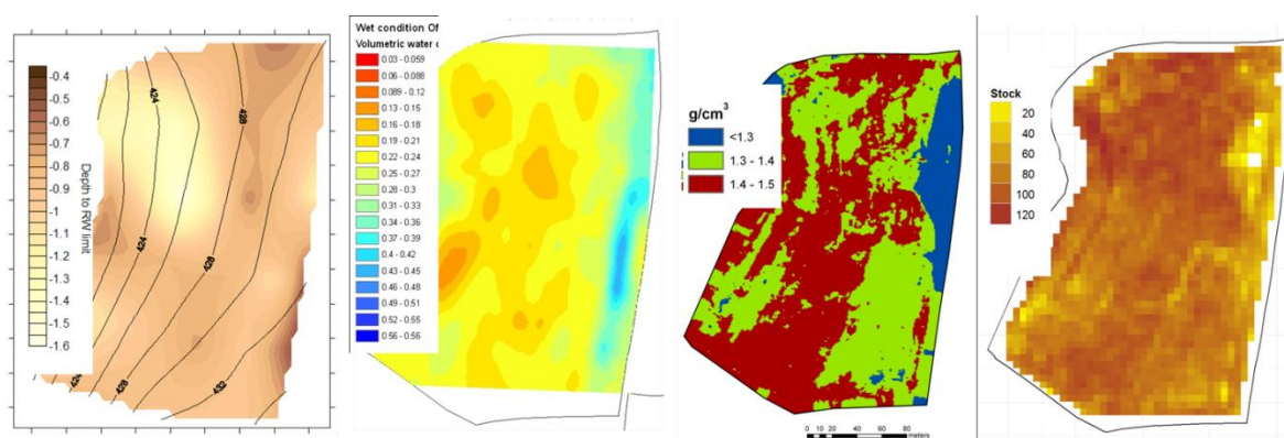
Fig. 3 – exemples de cartes de propriétés de sol obtenues sur le site du Luxembourg : épaisseur de sol, humidité, densité, stock de carbone.
